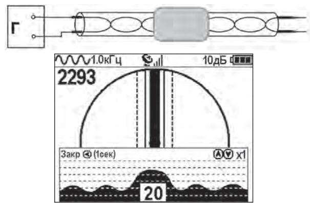
Рис.А.2 Муфта
